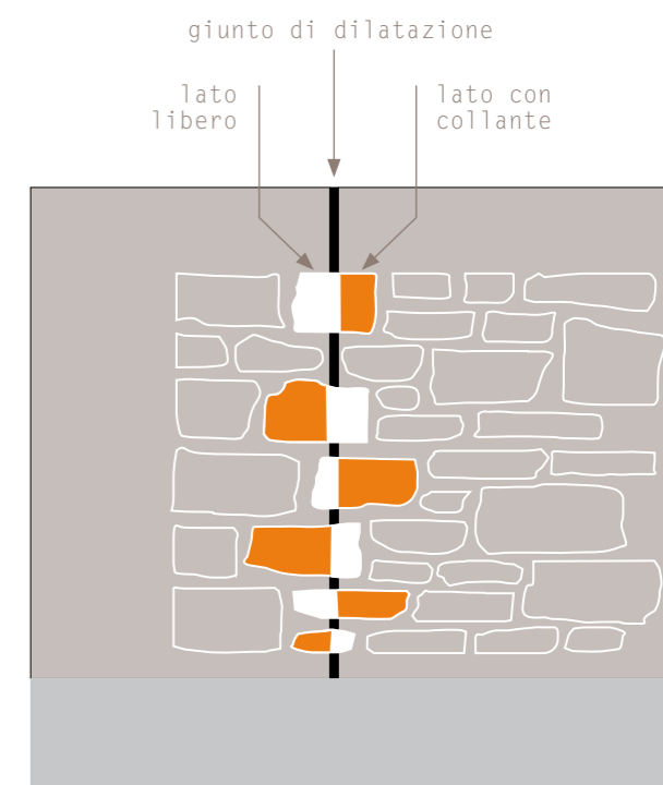
MASCHERATURA GIUNTI DI DILATAZIONE
