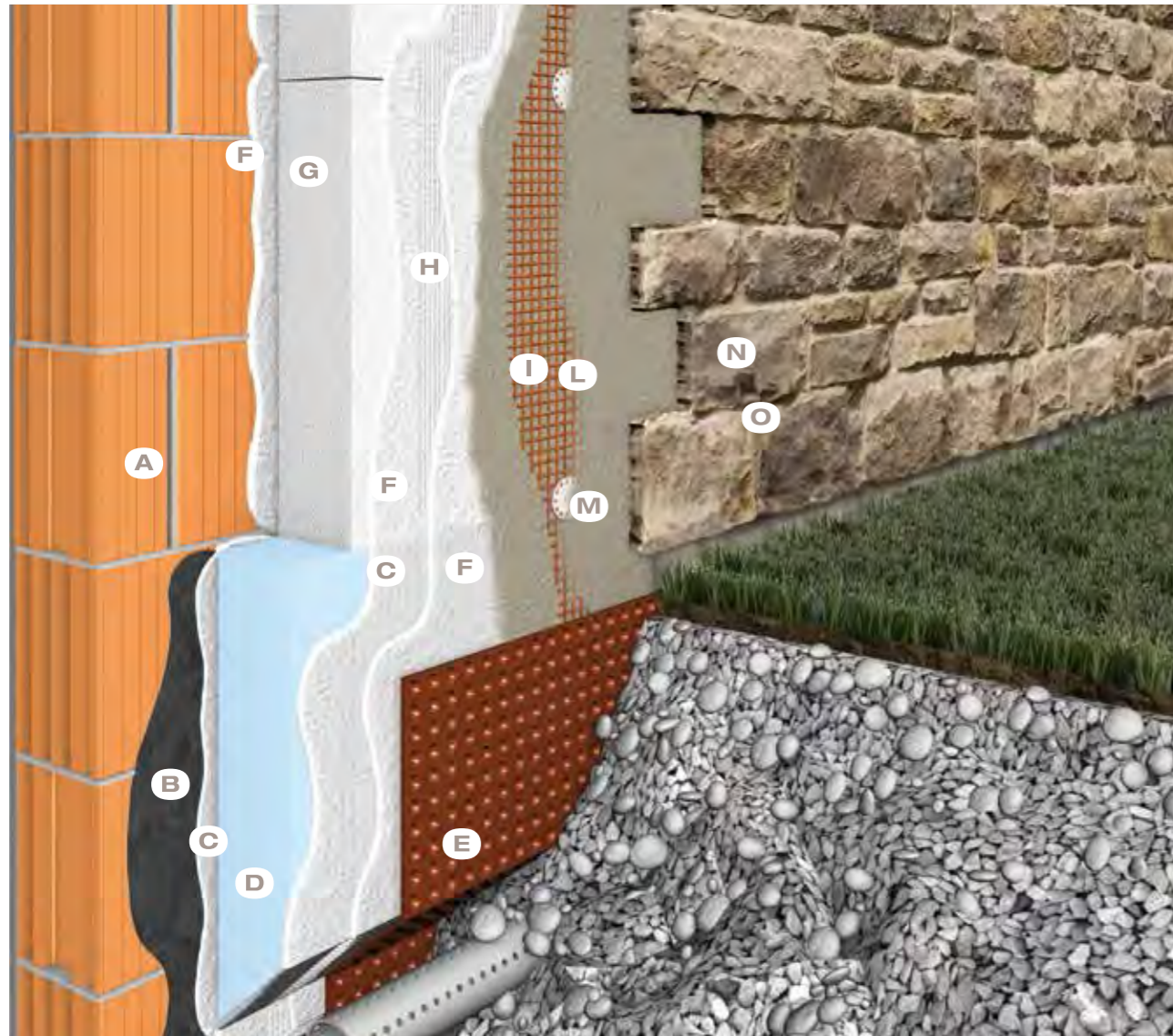
1.3 | schema generale e zoccolatura di partenza
